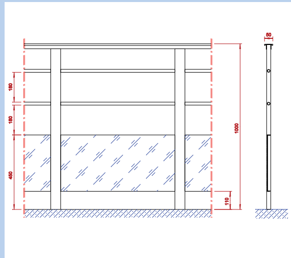
Borstwering volgens specifieke norm (Franse norm in het voorbeeld)
